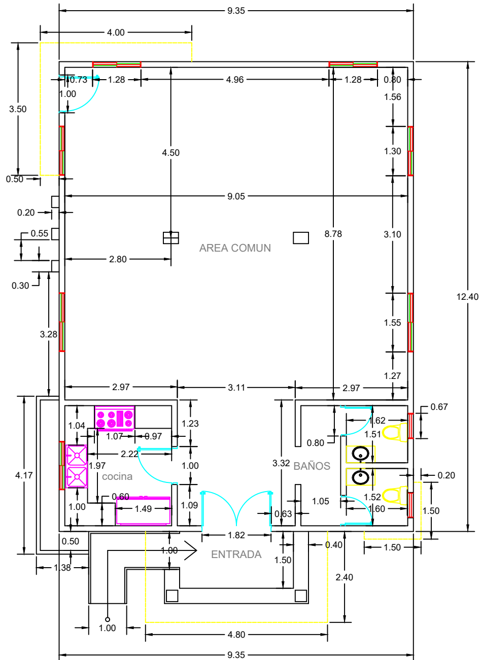
3 A PLANTA DIMENSIONADA 1:75
